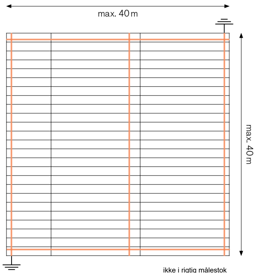
Fig. 2 – eksempel på ledende og dissipativ montering af noraplan ® ec/ec-baner til store arealer:
